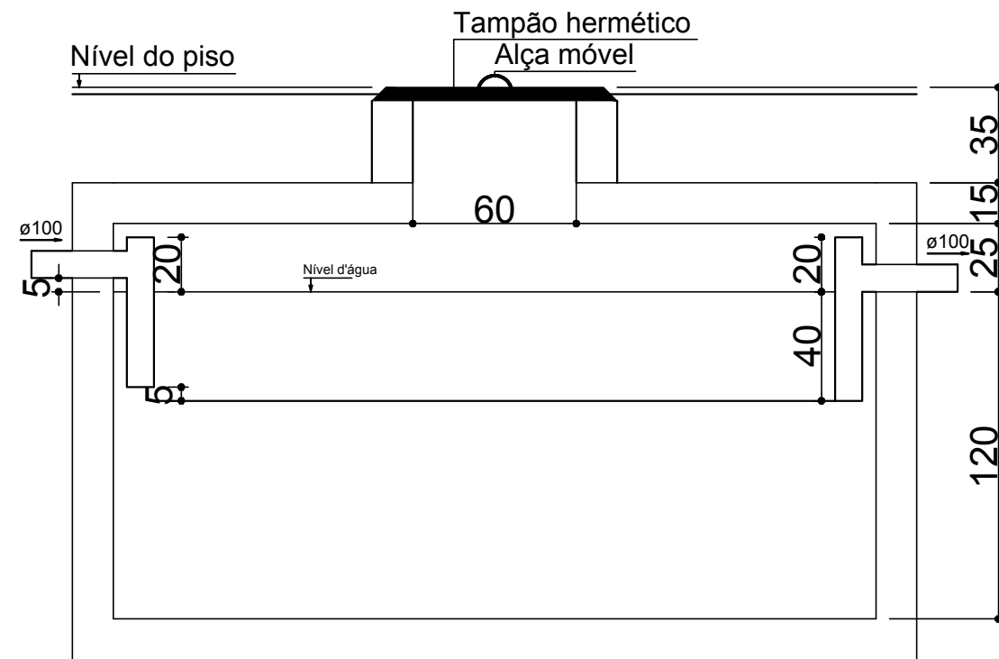
01 CORTE TANQUE SÉPTICO Esc. : 1 / 25
