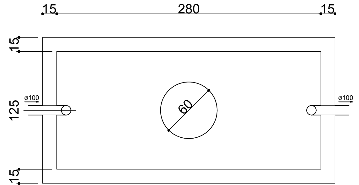
02 PLANTA TANQUE SÉPTICO Esc. : 1 / 25
