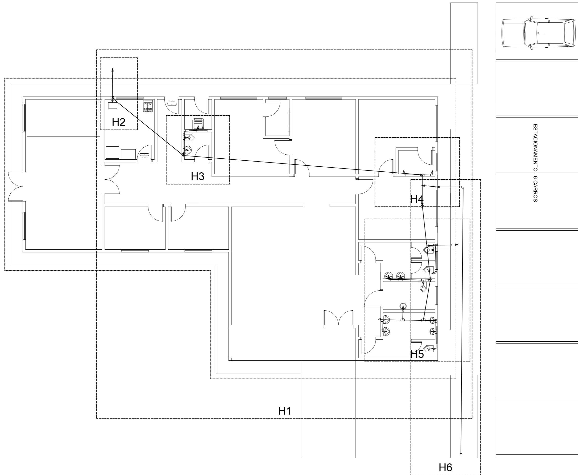
01 PLANTA DE INSTALAÇÃO HIDRÁULICA Esc.: 1 / 100
