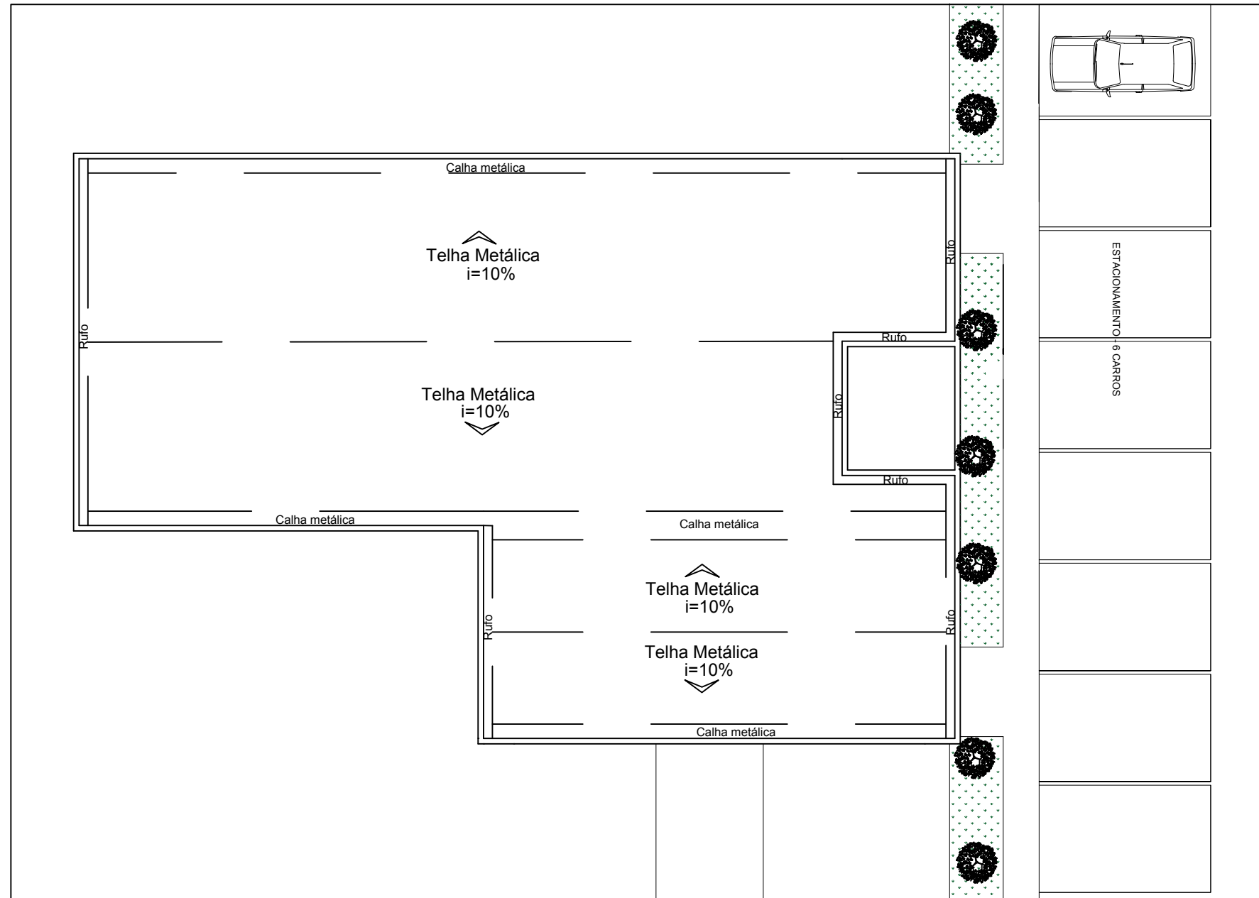
01 PLANTA DE COBERTURA Esc. : 1 / 150
